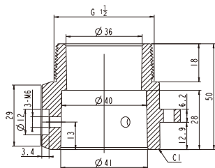
转接件规格
